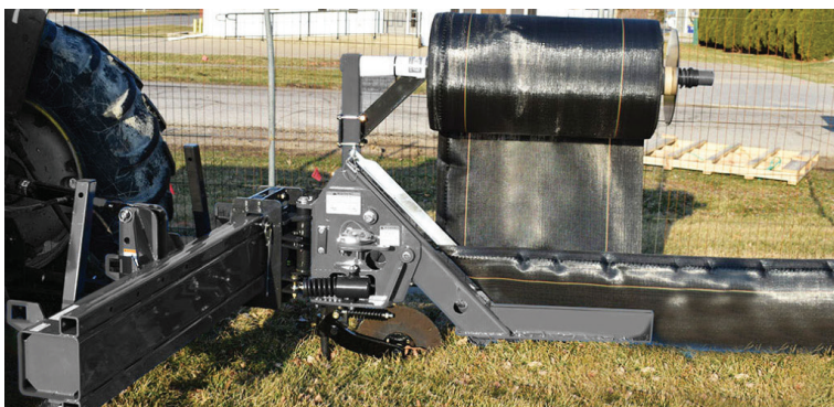
Side shift mount
